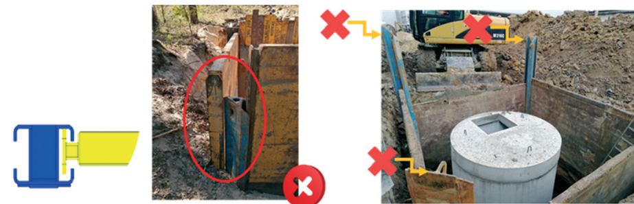
Rys. 10. Płyta płytowa obudowy systemowej nie została wsunięta w prowadnice słupa narożnego
